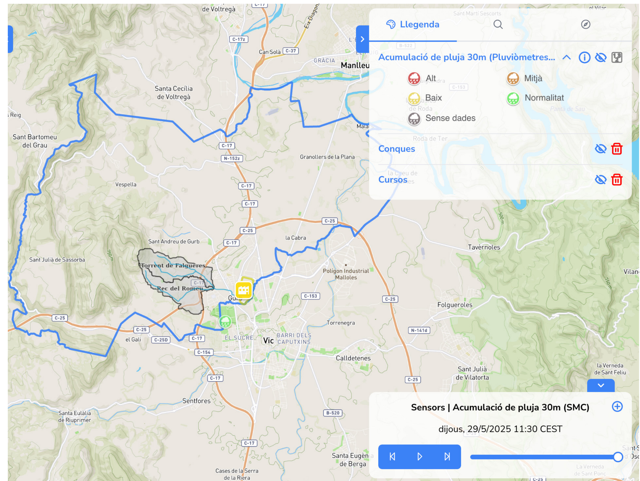
Sensors d'acumulació de pluja. Dades introduïdes a la plataforma Argos (HYDS, S.L) com a SAP
